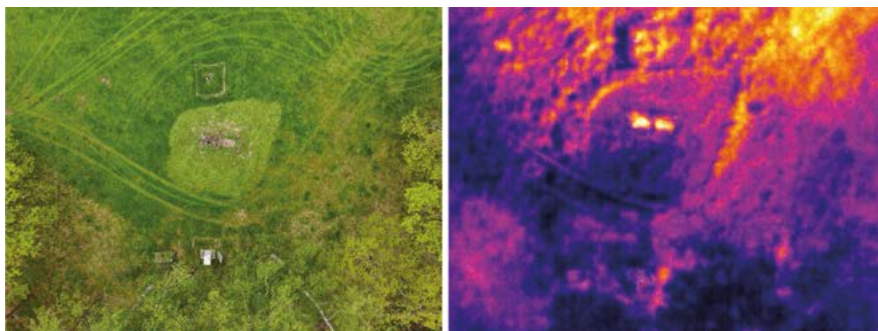
Obr. 12: Vizuální a termografický snímek kadáverů (vlevo 6 týdnů starý, vpravo 7 měsíců starý) z výšky 30 m
